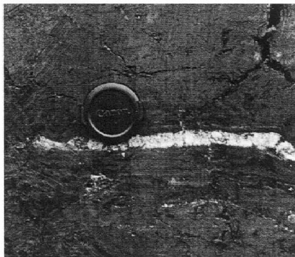
2: 島根大学構内遺跡橋縄手地区のアカホヤ火山灰層 レンズキャップの直径は約6cm
