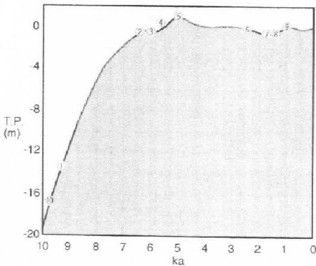
3: 島根県東部における完新世の海面変化
